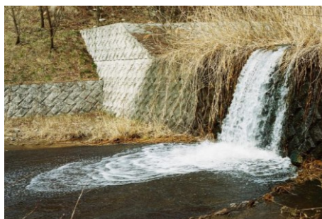
砂防ダム改修前（2008年）
